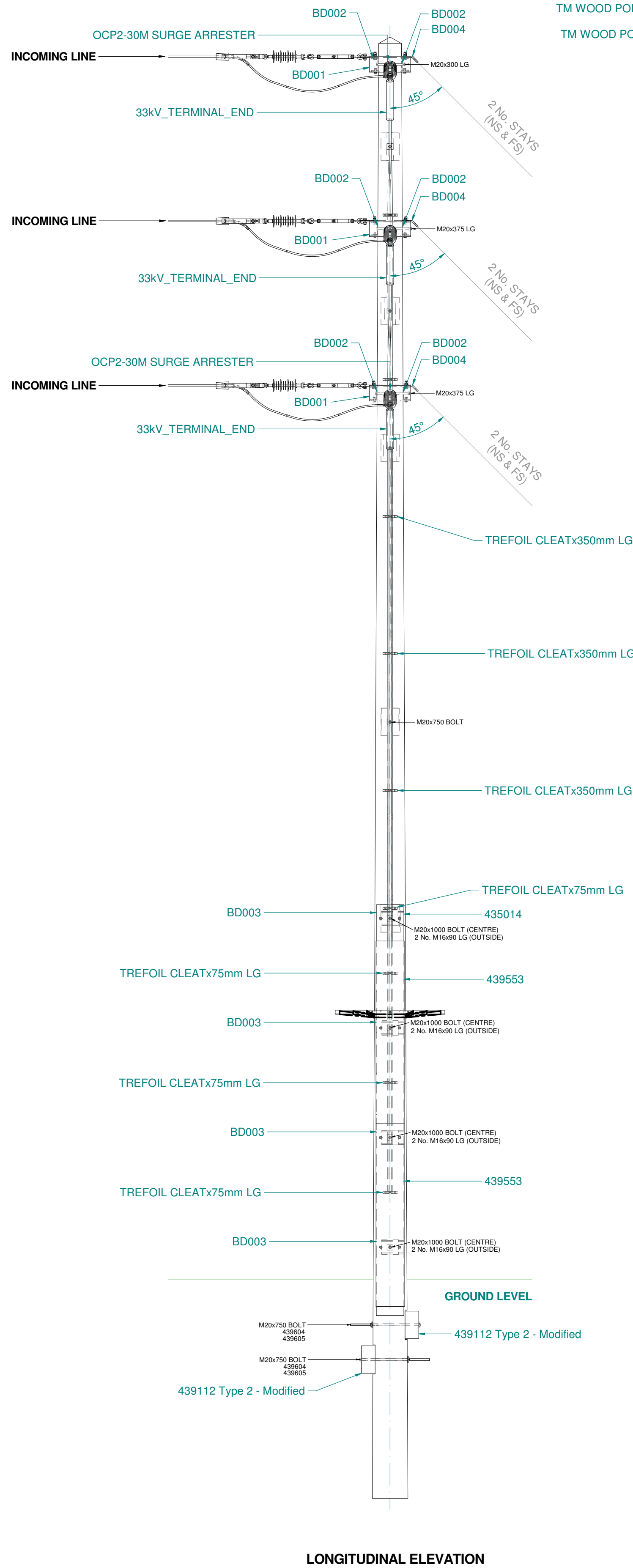
LONGITUDINAL ELEVATION
